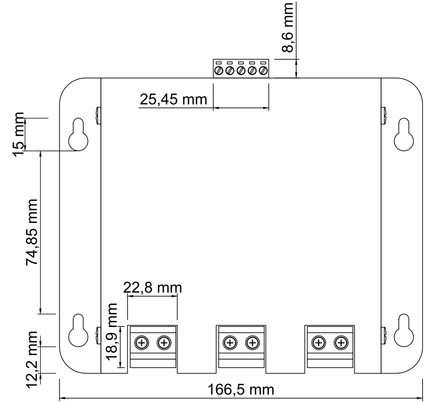
ÜST GÖRÜNÜŞ
