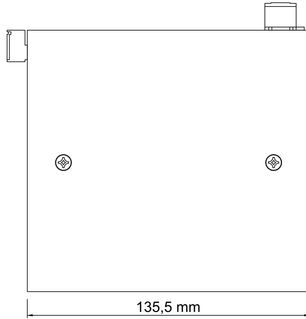
YAN GÖRÜNÜŞ
